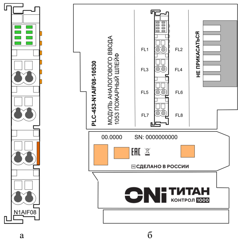
Рисунок 1 – Модуль N1AIF08 (а – вид спереди, б – вид справа)
