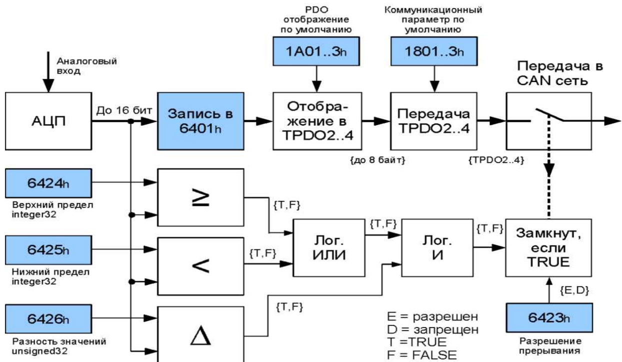
Рисунок 2 – Алгоритм работы модуля аналогового ввода
