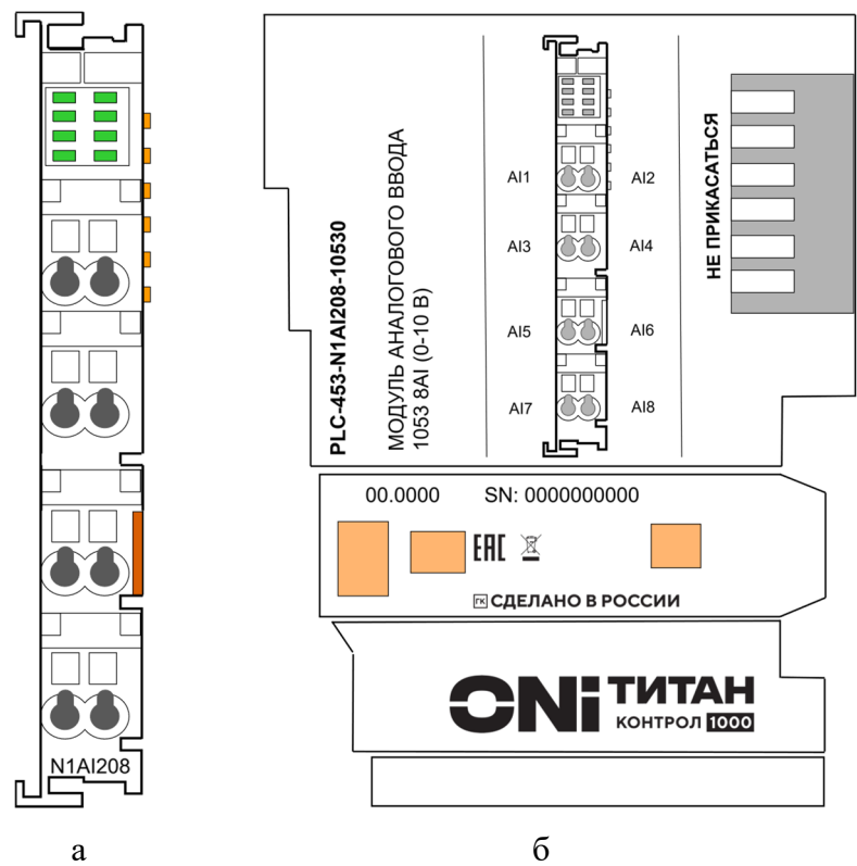
Рисунок 1 – Модуль N1AI208 (а – вид спереди, б – вид справа)
