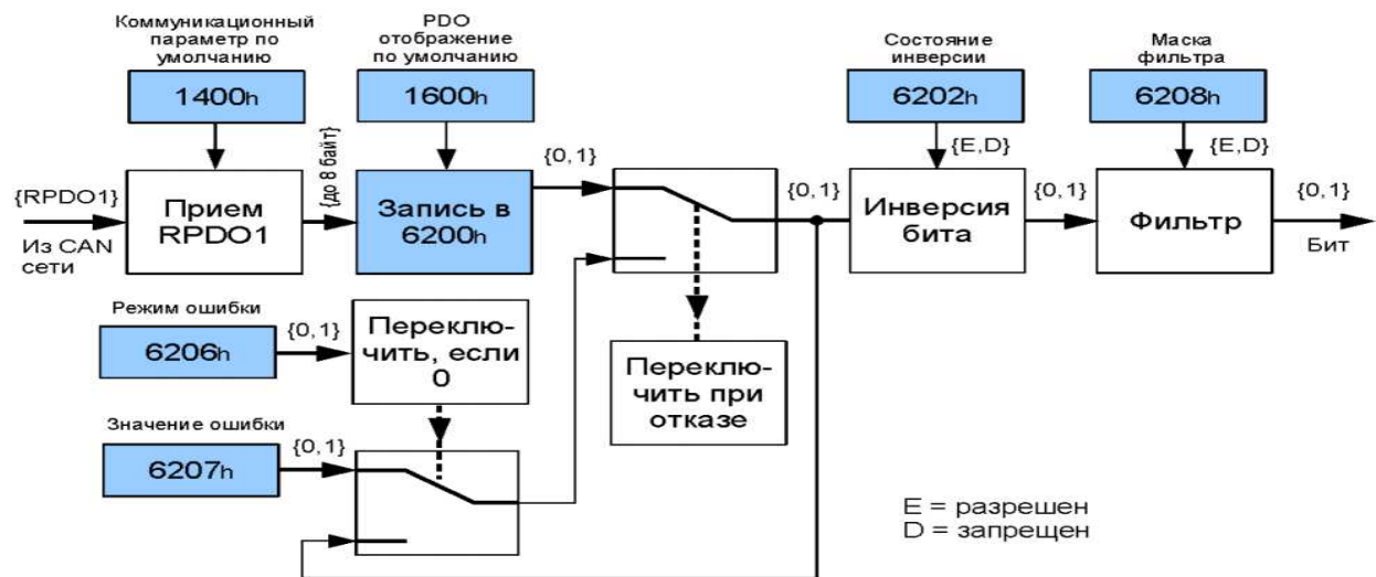
Рисунок 2 – Алгоритм работы модулей дискретного вывода
