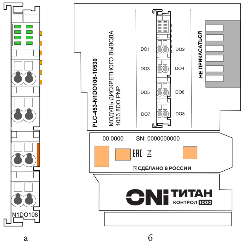
Рисунок 1 – Модуль N1DO108 (а – вид спереди, б – вид справа)
