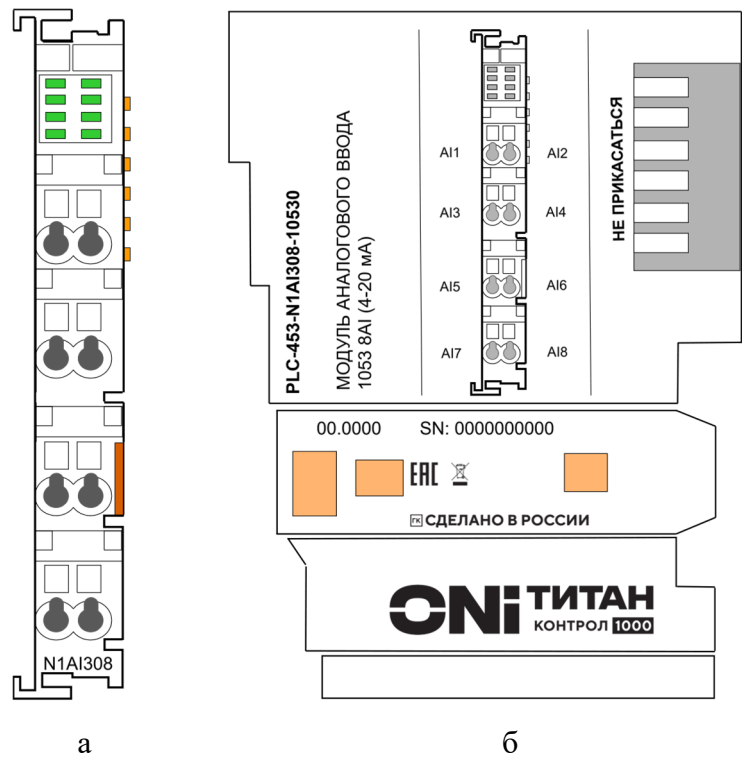
Рисунок 1 – Модуль N1AI308 (а – вид спереди, б – вид справа)
