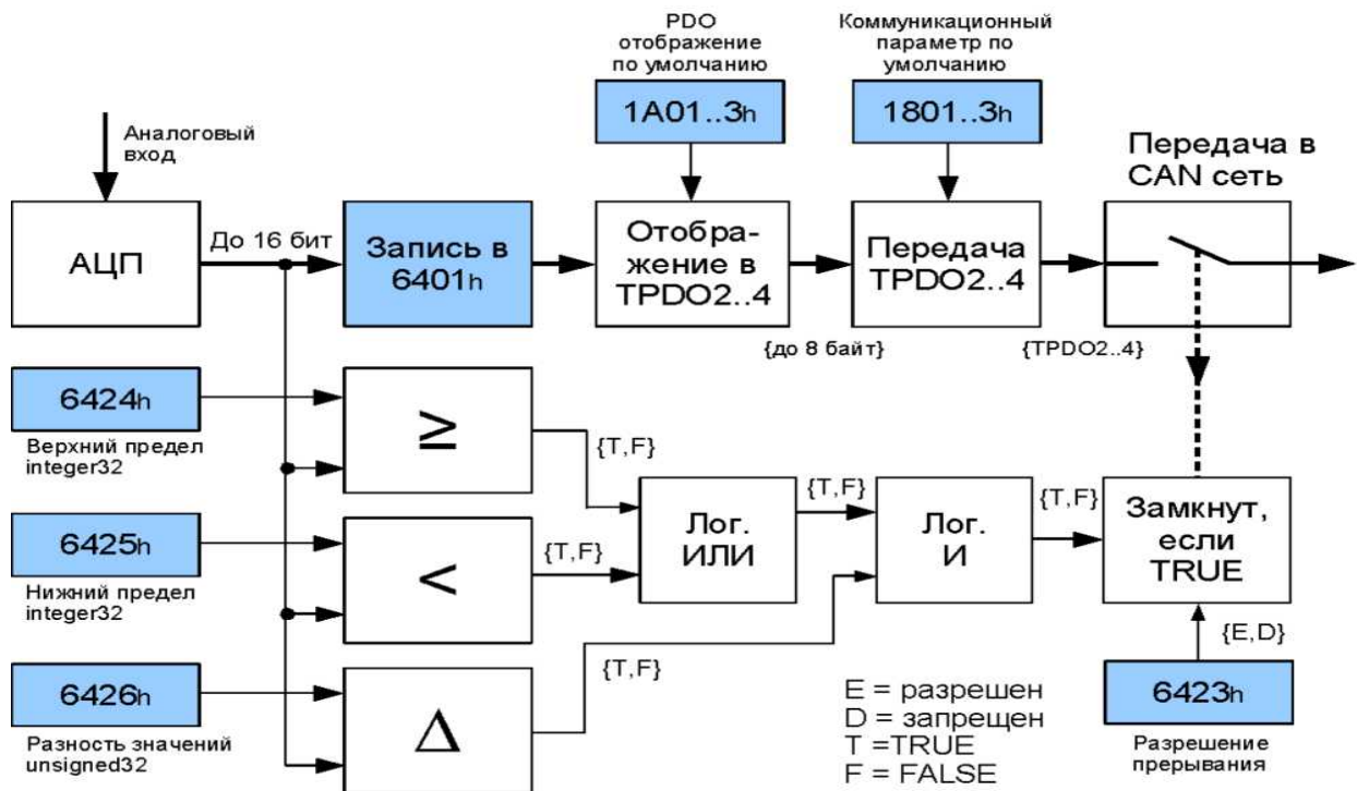
Рисунок 2 – Алгоритм работы модуля аналогового ввода
