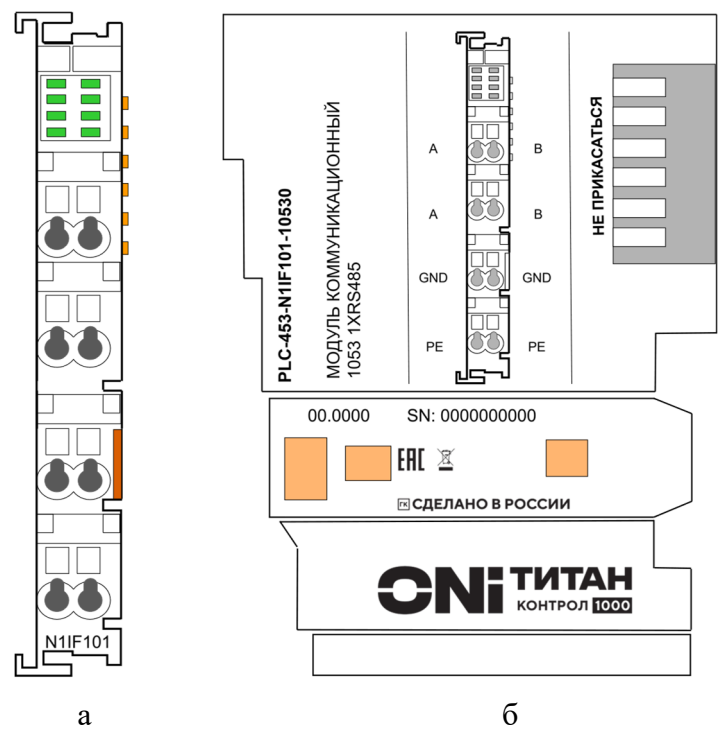
Рисунок 1 – Модуль N1IF101 (а – вид спереди, б – вид справа)
